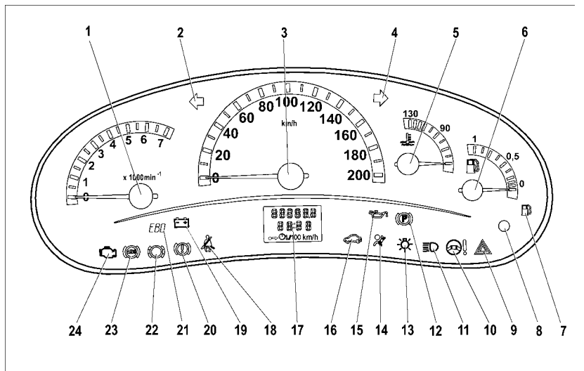
Рис. 29. Комбинация приборов
