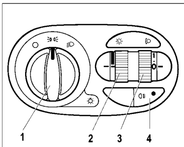
Рис. 31. Модуль управления светотехникой
